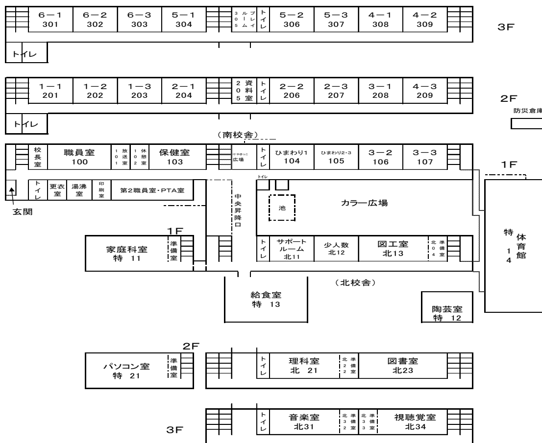
校舎平面図(教室等配置図) 令和6年度 四日市市立羽津北小学校
